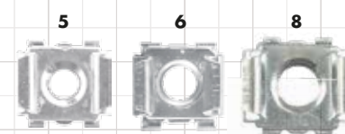
FAMILIA 00381 TUERCA ENJAULADA DE ACERO CINCADO (A2K). W-0381
