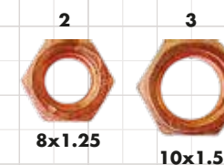
TUERCA HEXAGONAL DE ACERO BAÑADO EN COBRE. DIN 14441 CLASE 6
