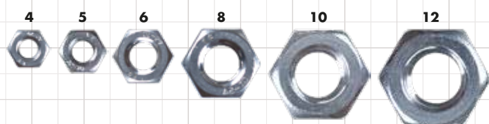
TUERCA HEXAGONAL DE ACERO INOXIDABLE T-304 (A2-70). DIN 934 (ISO 4032)
